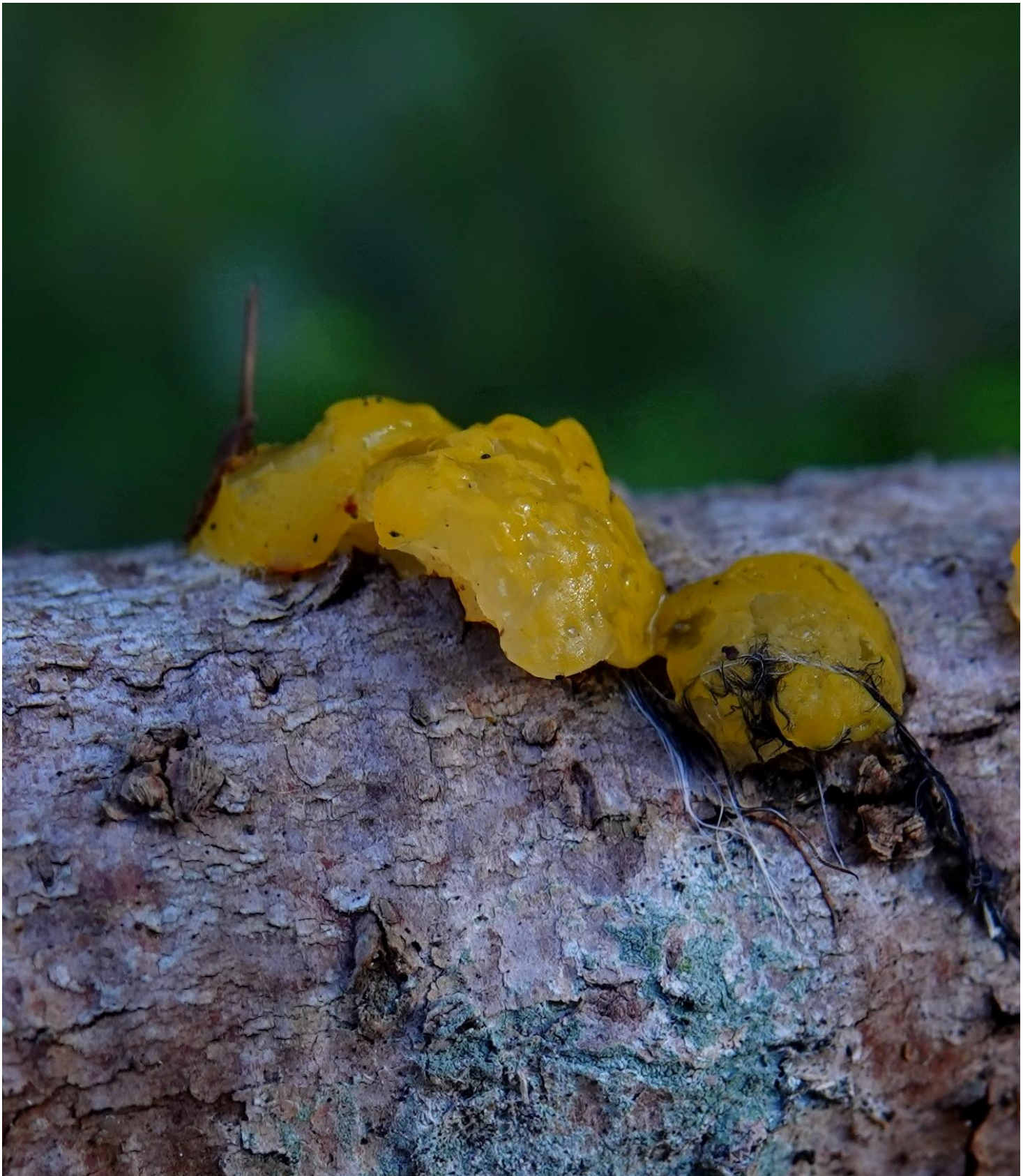
Dacrymyces stillatus Nees : Fr., 1817 Trémelle déliquescence - Protoclavaire déliquescence Dacrymycetales - Dacrymycetaceae
